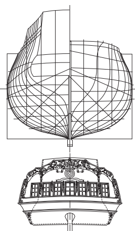
▼ Plan de l'Iris-Hancock, à son arrivée en Angleterre NMM Greenwich. A son arrivée à Greenwich, l'Hancock est rebaptisée Iris.
