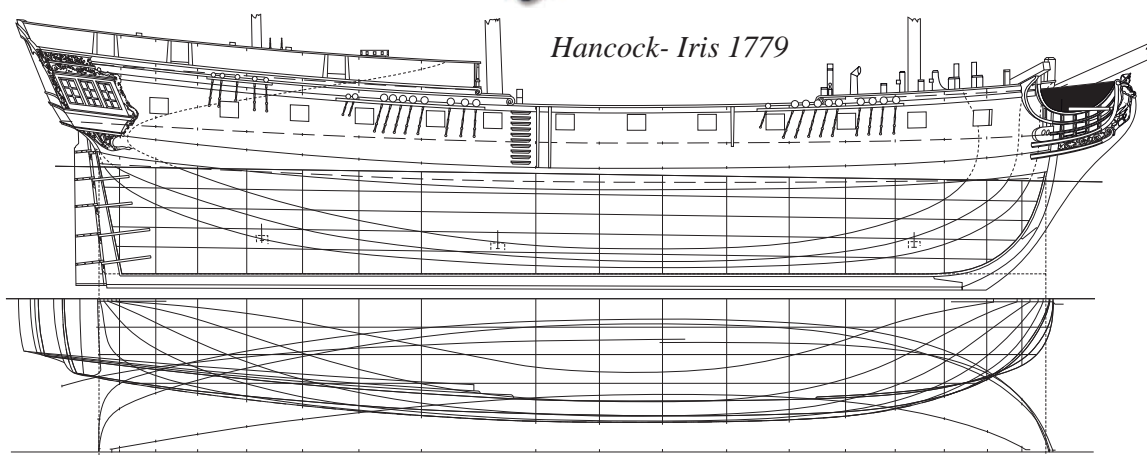
▼ Plan de l'Iris-Hancock, à son arrivée en Angleterre NMM Greenwich. A son arrivée à Greenwich, l'Hancock est rebaptisée Iris.
