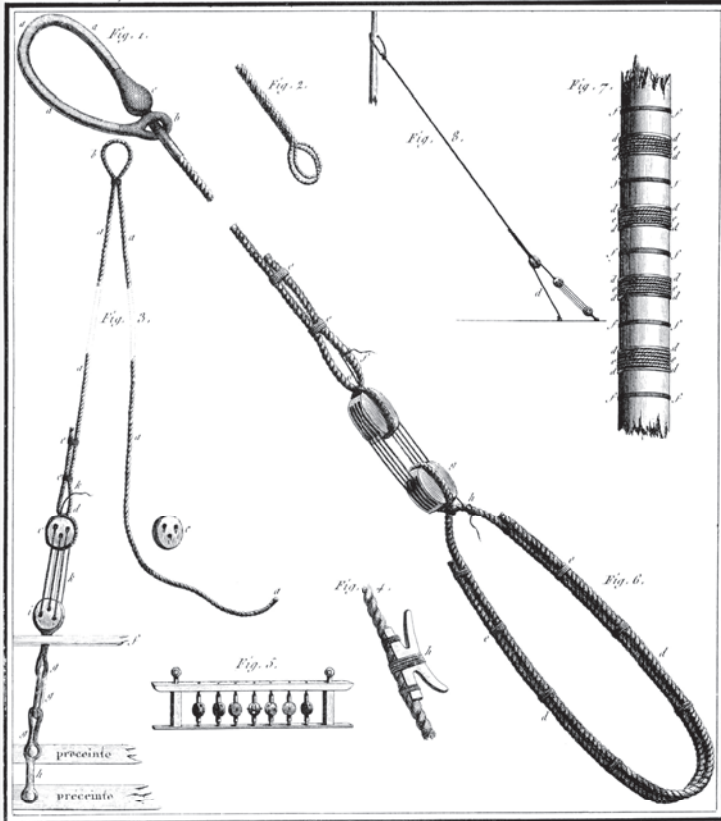
Pour le 2. e Livre Chapitre 1. er Art. 1. et 3. du Traité du Gréement
