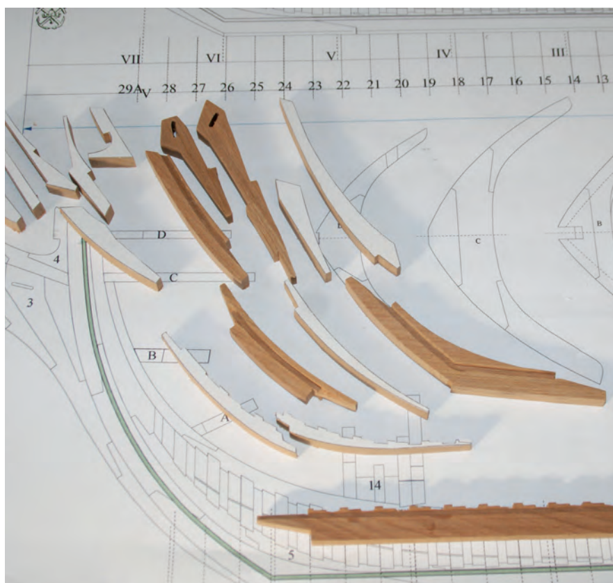
Photo 6 - Pièces de l'ossature longitudinale semi ouvrées. quille, étrave et contre-quille.
